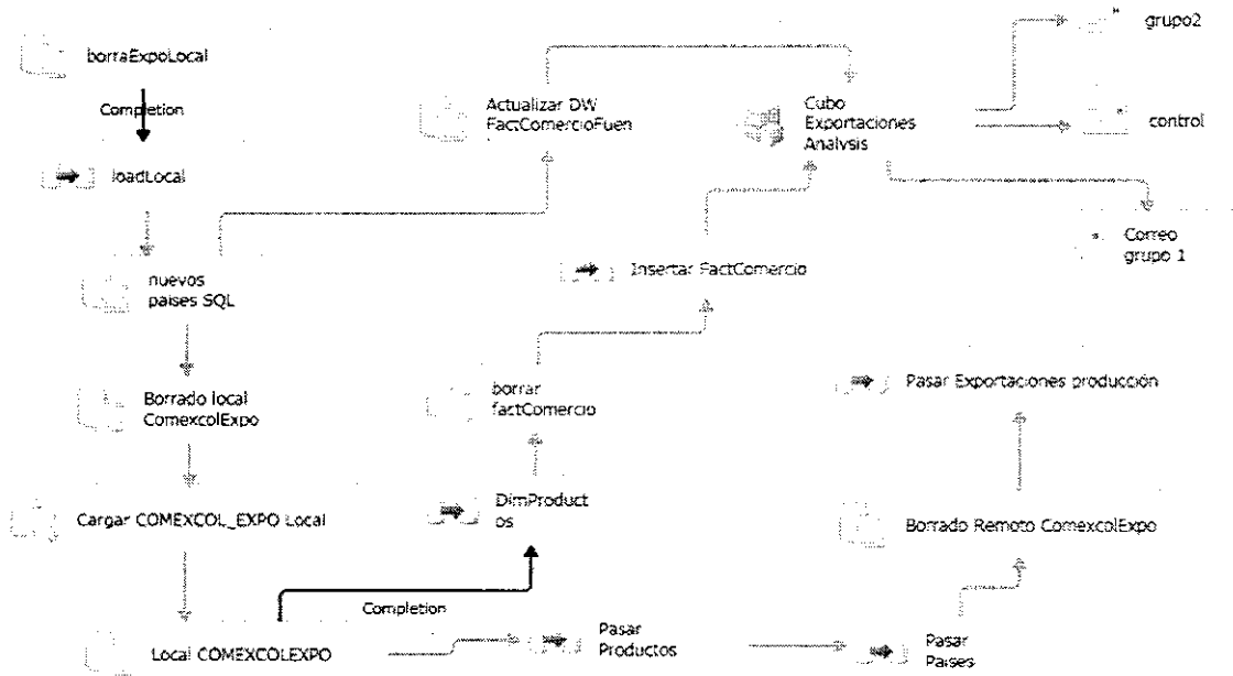
Figura 5. Cargar Exportaciones
