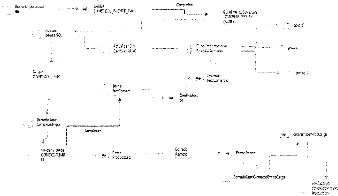
Figura 4. Cargar importaciones
