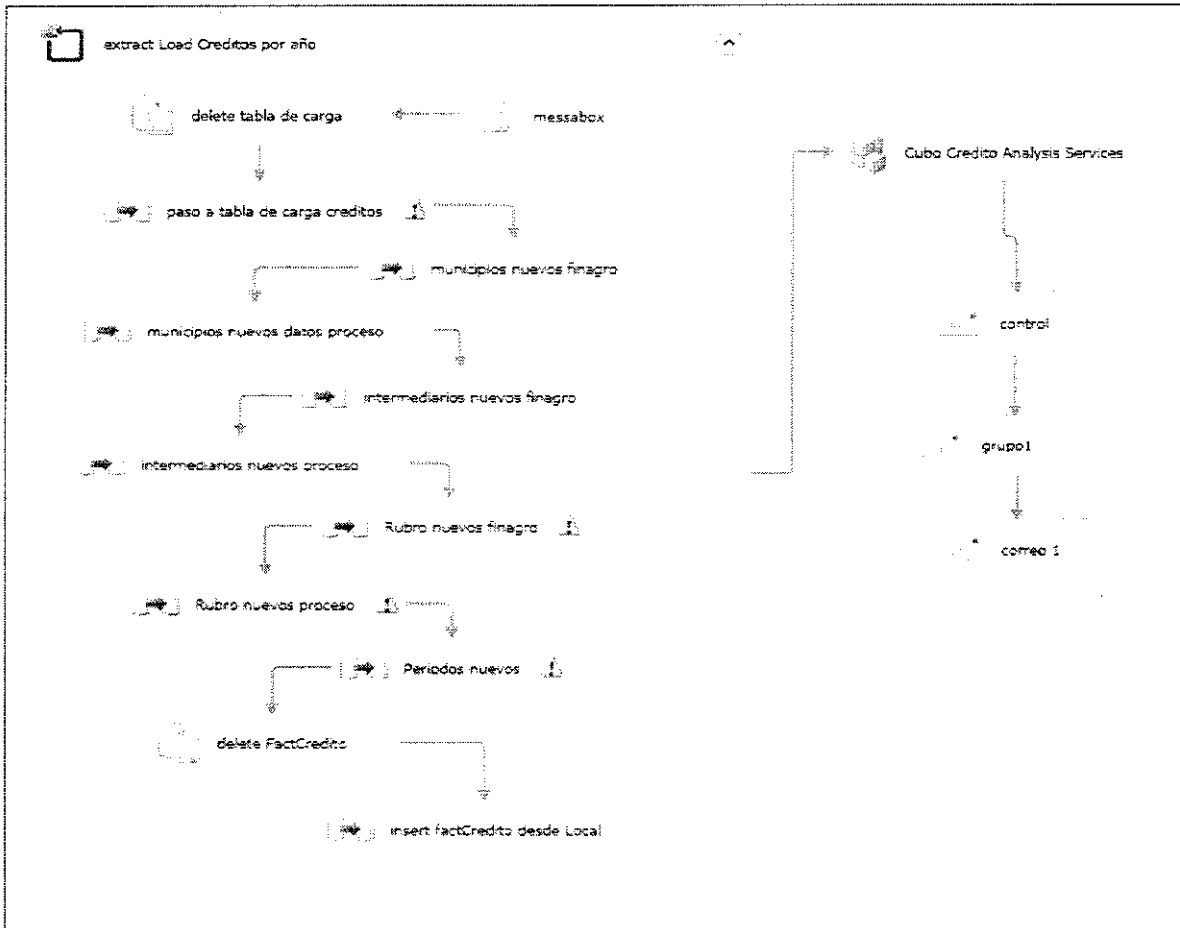
Figura 9. creditoLoadFactTable.dtsx
