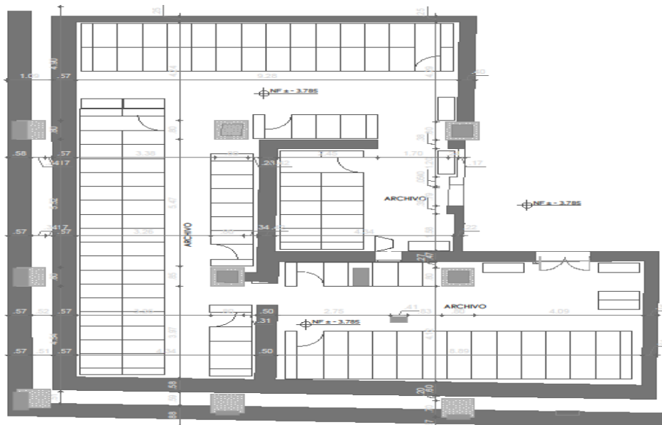
PLANTA ARCHIVO AREA DE INTERVENCION SOTANO ESC. 1 : 50
