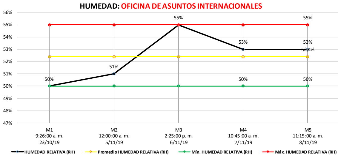
Gráfico 15 Humedad oficina de asuntos internacionales
