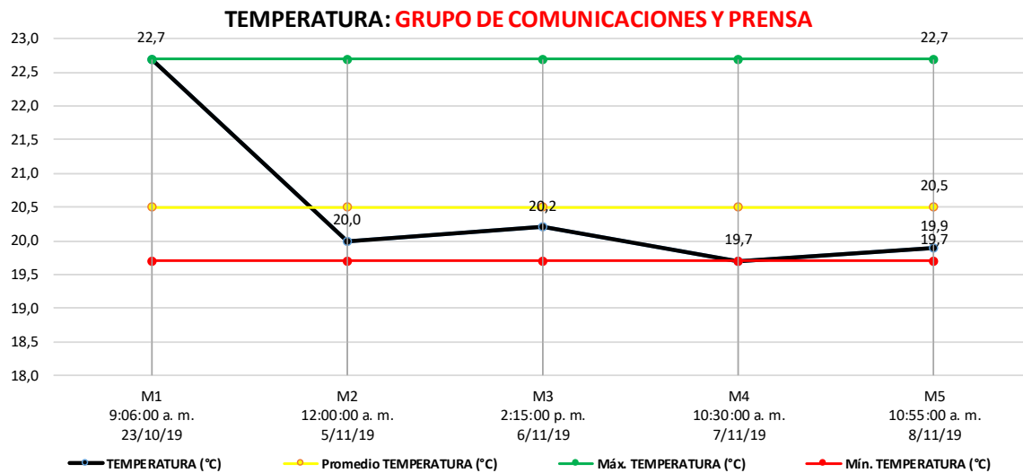
Gráfico 10 Temperatura grupo de comunicaciones y prensa
