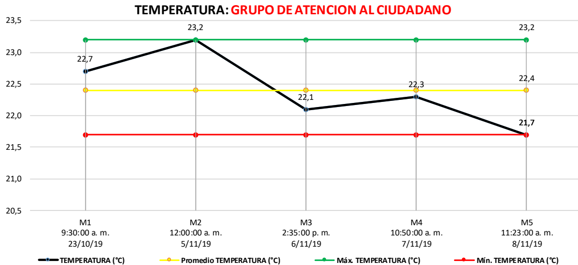
Gráfico 19 Temperatura grupo de atención al ciudadano
