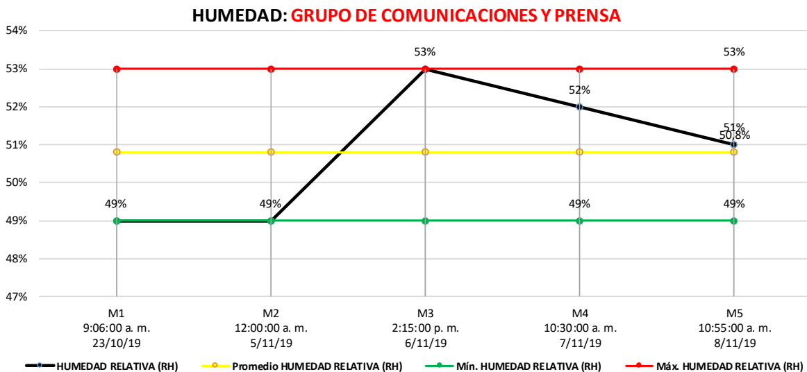
Gráfico 9 Humedad grupo de comunicaciones y prensa
