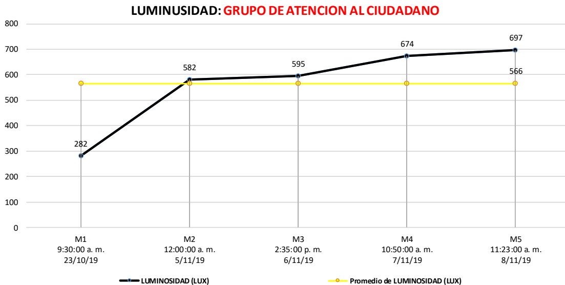
Gráfico 20 Luminosidad grupo de atención al ciudadano
