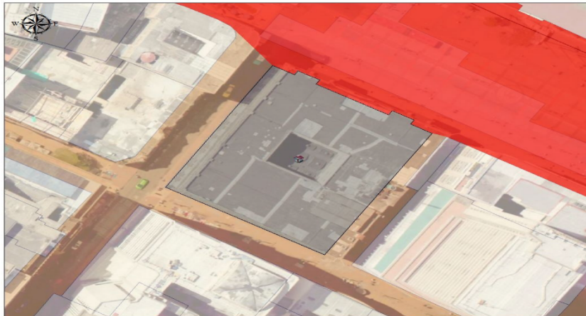
Ilustración 3 Zona de reserva vial, según Decreto #190 de 2.004 POT
