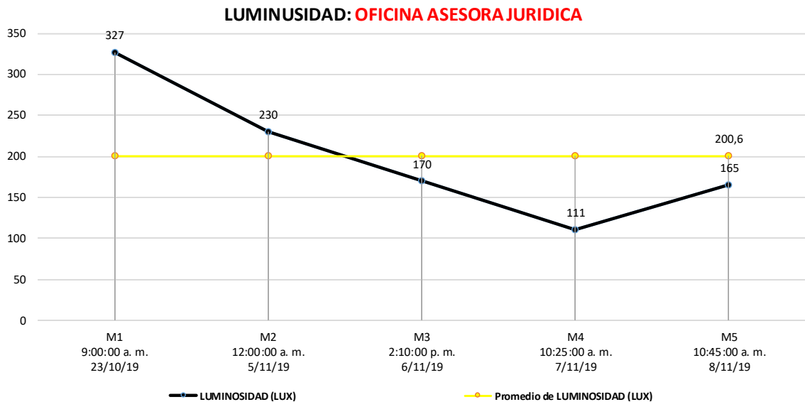
Gráfico 8 Luminosidad oficina asesora jurídica
