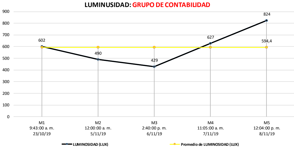
Gráfico 29 Luminosidad grupo de contabilidad
