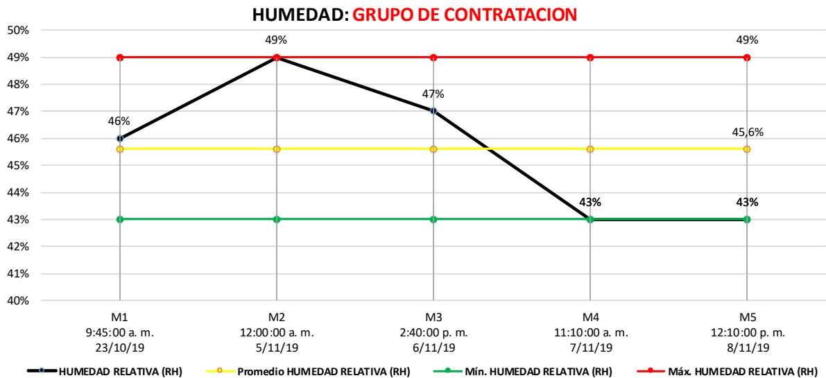
Gráfico 30 Humedad grupo de contratación
