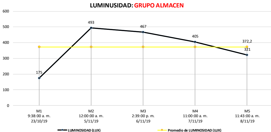
Gráfico 26 Luminosidad grupo de almacén
