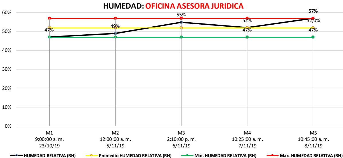
Gráfico 6 Humedad oficina asesora jurídica
