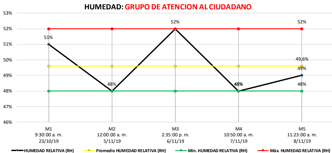
Gráfico 18 Humedad grupo de atención al ciudadano
