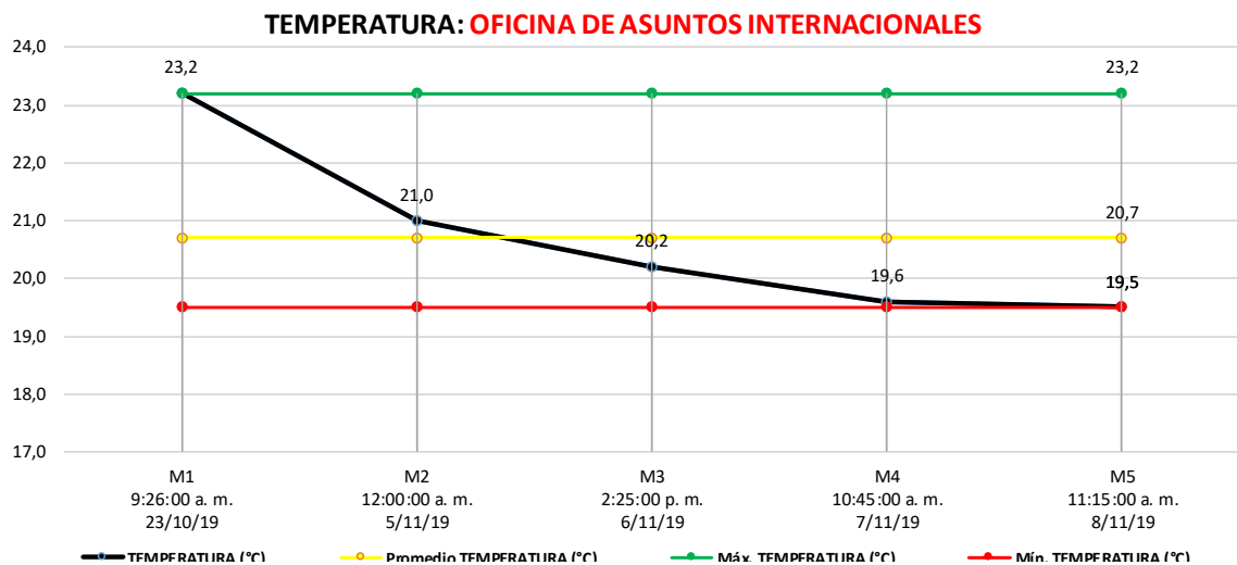
Gráfico 16 Temperatura oficina de asuntos internacionales
